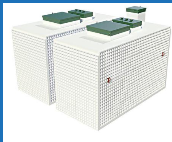
ТОПАС 150 Хүний тоо:150 Хүчин чадал:24000л Цахилгаан:23,6квт Жин:2045кг 3200/4700/3000мм
