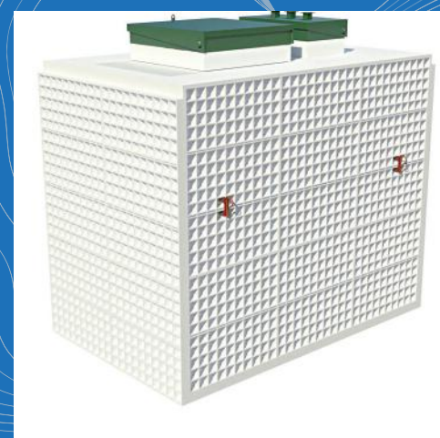
ТОПАС 50 Хүний тоо:50 Хүчин чадал:9000л Цахилгаан:8,0 квт Жин:1235кг 3300/2200/3000мм
